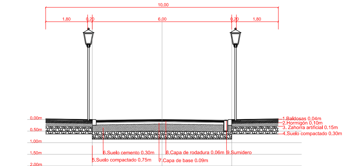
Sección transversal calle tipo 2.
