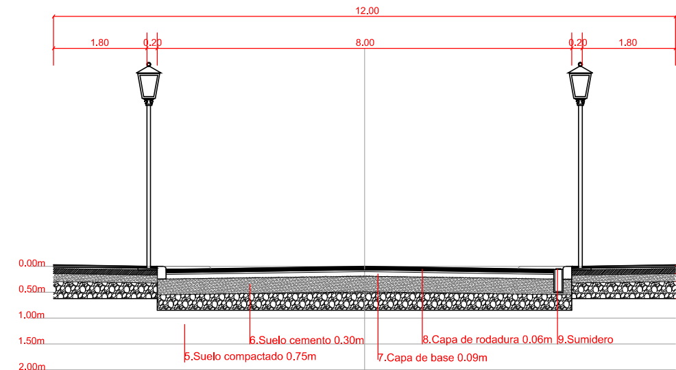
Sección transversal calle tipo 1.
