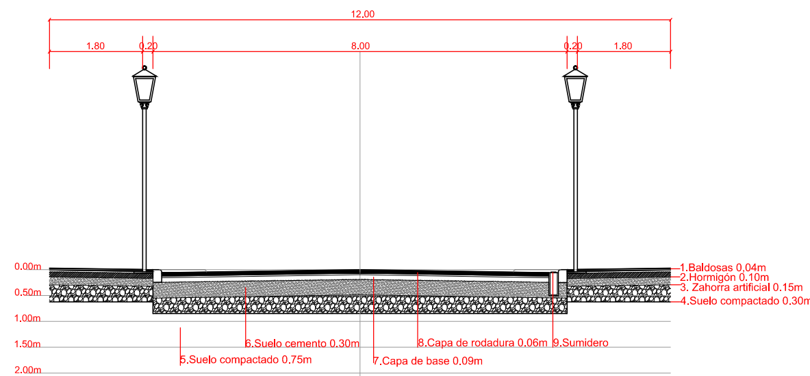
Sección transversal calle tipo 1.
