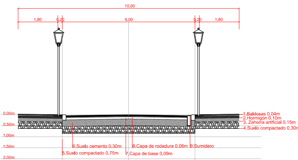
Sección transversal calle tipo 2.
